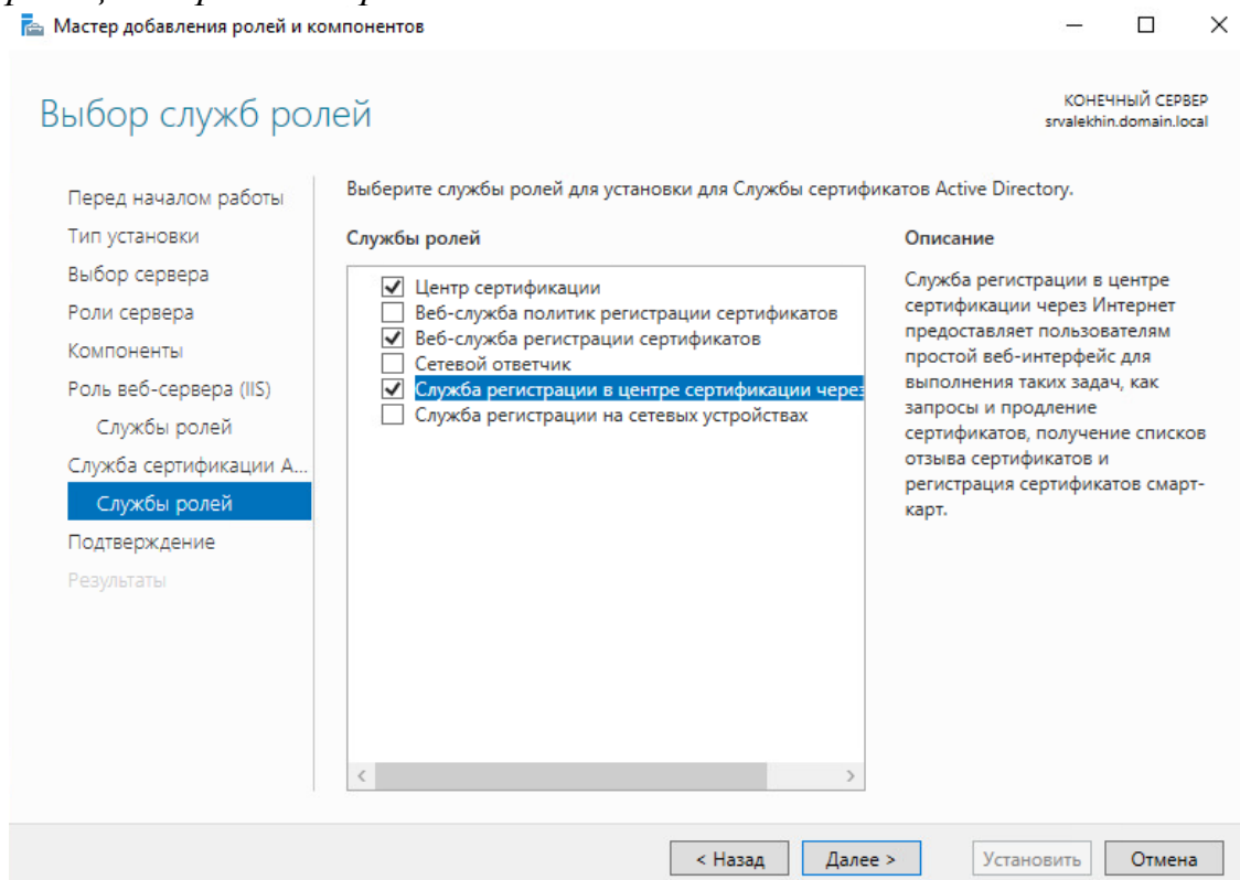
Рис. 2 Роли службы сертификации.
